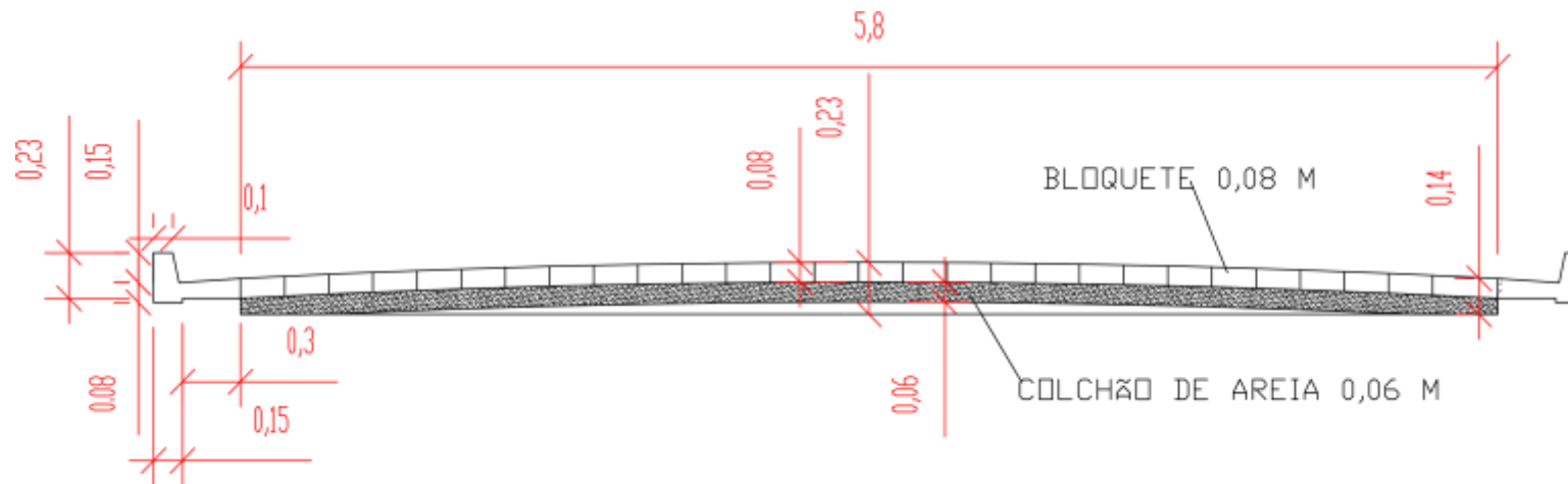
SEÇÃO S/ESCALA
