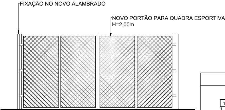
GRAMADO DO CAMPO DETALHE PORTÃO SEM ESCALA
