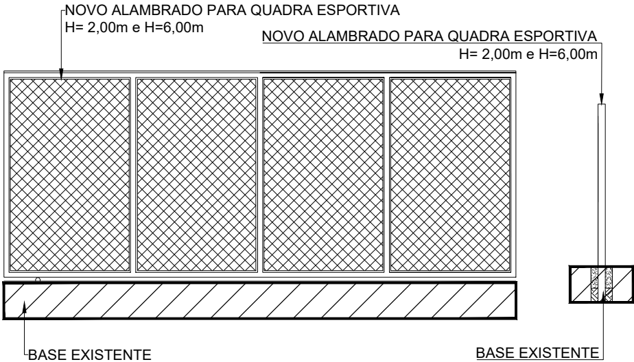
CORTE AA - NOVO ALAMBRADO SEM ESCALA
