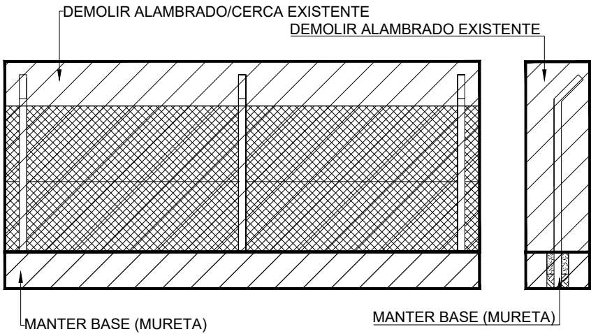
CORTE AA - ATUAL SEM ESCALA
